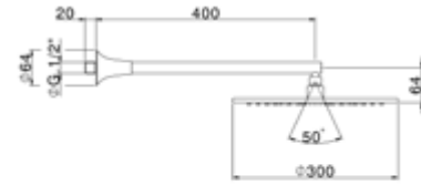
VI 013190 Braccio e Soffione Doccia Shower Arm & Head Bras et Tête de Douche
