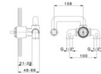
ZA 025510 Parte Incasso Monocomando Lavabo Basin Mixer Concealed Part Partie Encastrée Mitigeur Lavabo
