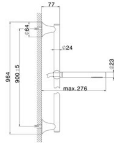
VI 003111 Completo Doccia Saliscendi 90 cm 90 cm Slide Rail Shower Set Ensemble Barre de Douche 90 cm
