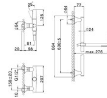
VI 000464 Completo Monocomando Doccia Shower Mixer Set Ensemble Mitigeur Douche
