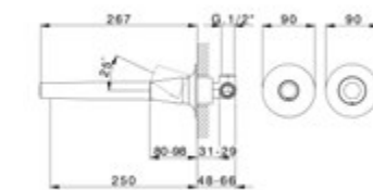
VI 002471 Completo Monocomando Lavabo Parte Incasso + Parte Esterna Basin Mixer Set Concealed Part + Exposed Part Ensemble Mitigeur Lavabo Partie Encastrée + Partie Apparente
