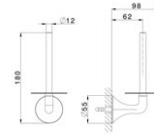
VI 090410 Porta Rotolo Roll Holder Porte-Papier
