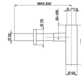
ZA 004070 Sifone Siphon Siphon
