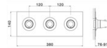
VI 01R200 Parte Esterna Termostatico 2 Funzioni 2-Function Thermo Exposed Part Partie Décor Thermo 2 Fonctions
