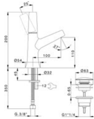
VI 000514 Monocomando Lavabo Basin Mixer Mitigeur Lavabo
