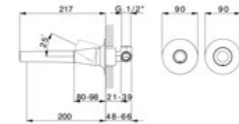
VI 002470 Completo Monocomando Lavabo Parte Incasso + Parte Esterna Basin Mixer Set Concealed Part + Exposed Part Ensemble Mitigeur Lavabo Partie Encastrée + Partie Apparente
