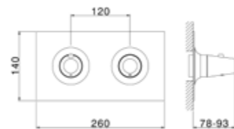
VI 019140 Parte Esterna Termostatico 2 Uscite 2-Outlet Thermo Exposed Part Partie Décor Thermo 2 Sorties
