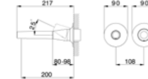
VI 005510 Parte Esterna Monocomando Lavabo Basin Mixer Exposed Part Partie Apparente Mitigeur Lavabo
