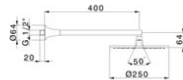
VI 013191 Braccio e Soffione Doccia Shower Arm & Head Bras et Tête de Douche
