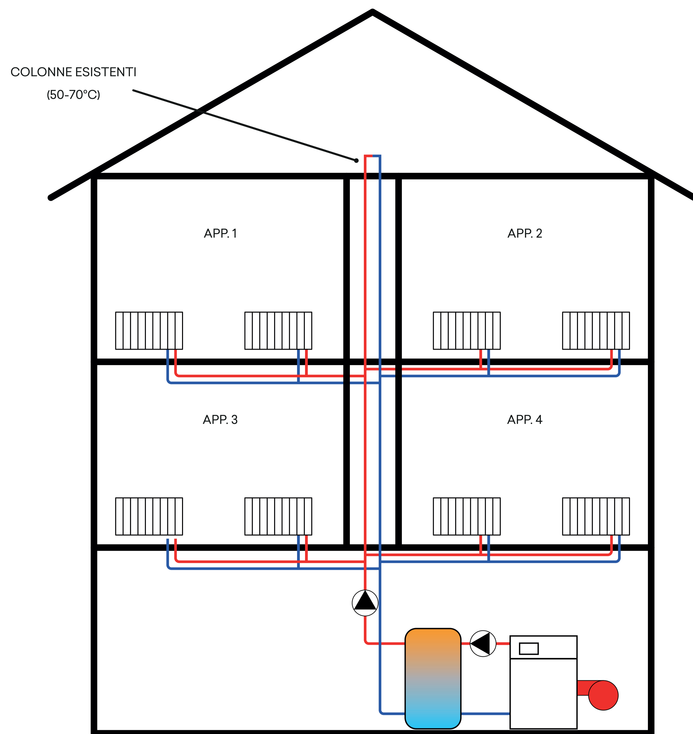
IMPIANTO ESISTENTE
