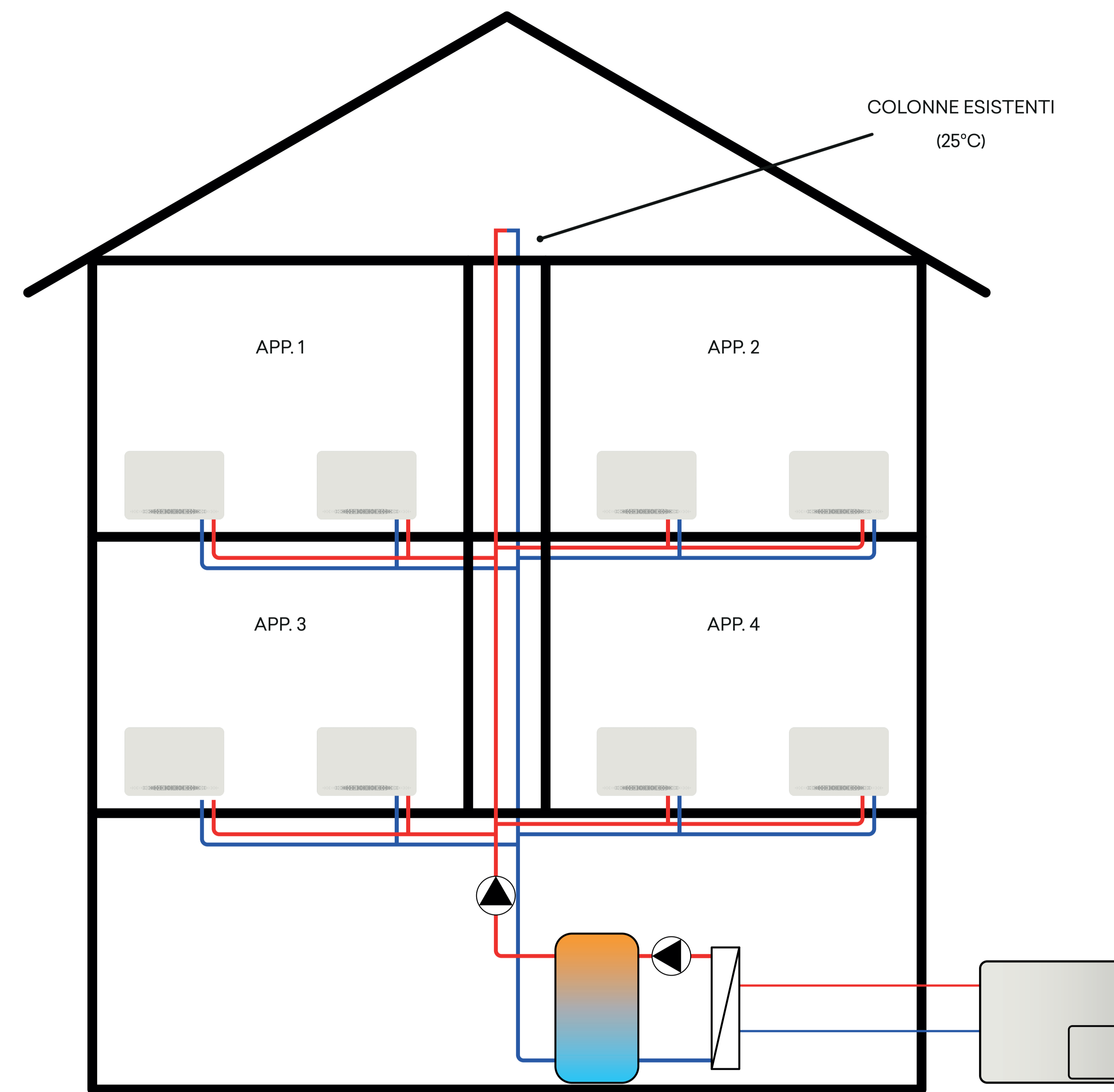
IMPIANTO RIQUALIFICATO
